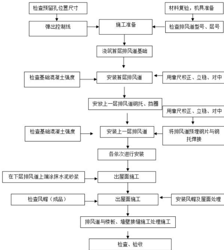
附图：排风道安装施工工艺流程图
